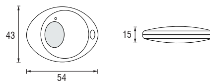
Ⓑ Telecomando IR IR Remote control / IR Fernsteuerung
